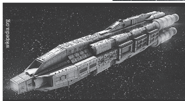
Вверху: примерно так, по расчетам, выглядит астероид. Внизу: Оумуамуа вполне может быть и вот таким длинным космическим кораблем.
